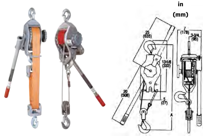
C-Series Pullers
